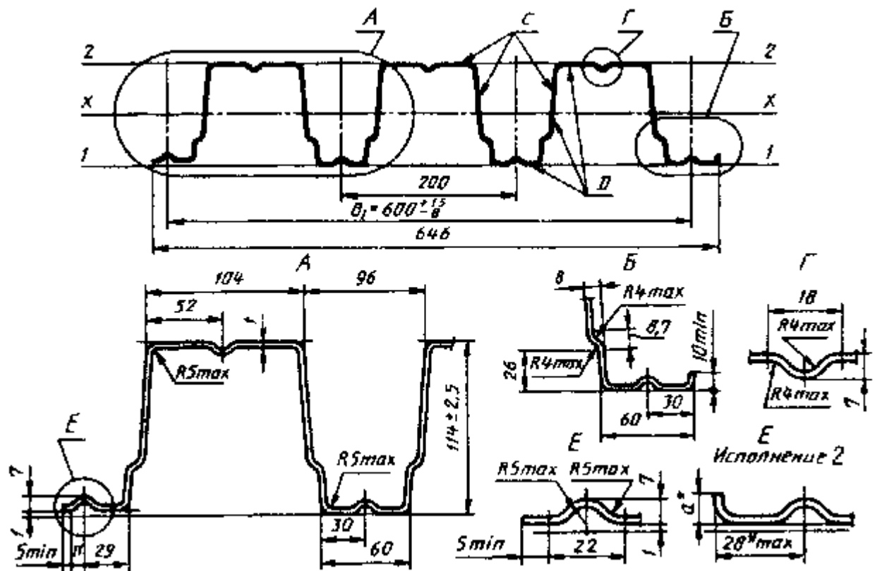
Рисунок 3 - Профилированный лист типа Н высотой 114 мм, шириной 600 мм
