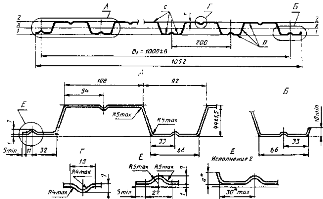
Рисунок 6 - Профилированный лист типа HC высотой 44 мм
