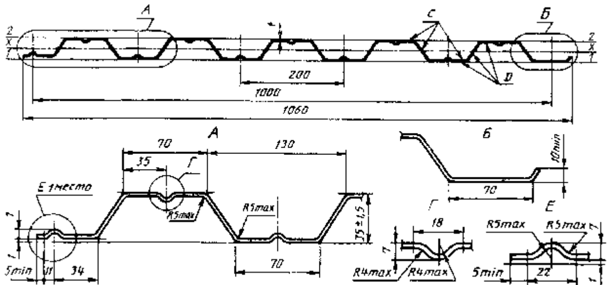
Рисунок 5 - Профилированный лист типа HC высотой 35 мм
